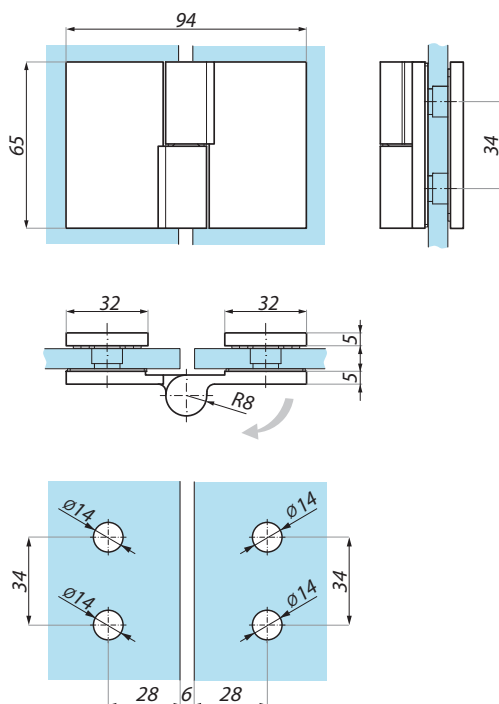
Príprava skla Glass preparation
