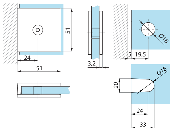
Príprava skla Glass preparation
