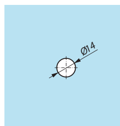
Príprava skla Glass preparation
